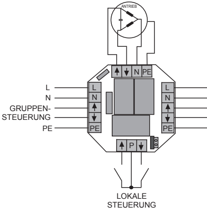
Abb. 1 Anschlussschema des SIR-Steuergeräts mit Jalousieschalter
