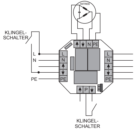
Abb. 2 Anschlussschema des SIR-Steuergeräts mit Klingelschalter
